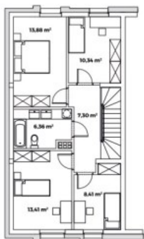
PIĘTRO
